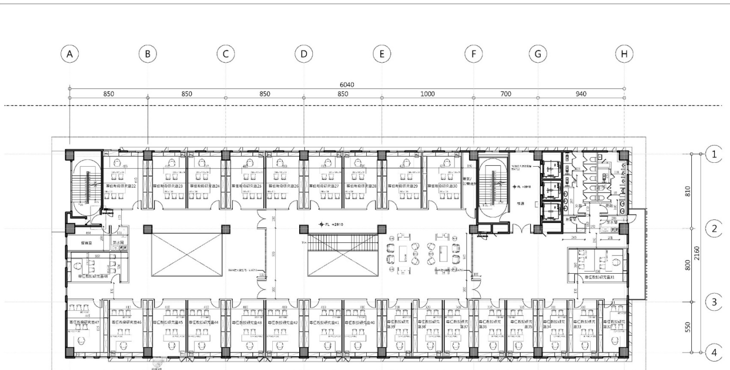
八樓平面圖 A3=1/200 A1=1/100 樓地板面積 1366.703 m 2
