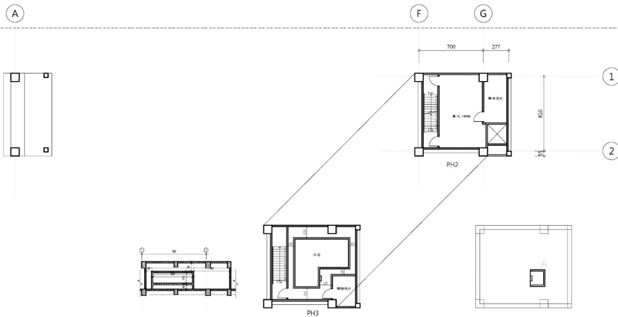
屋突二、三層平面圖
